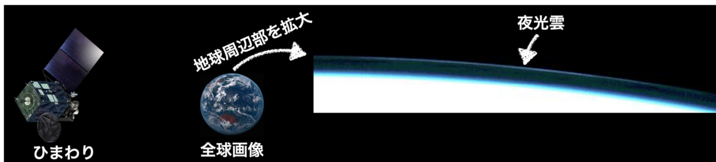
図 1: 静止軌道衛星ひまわりによる夜光雲の観測
